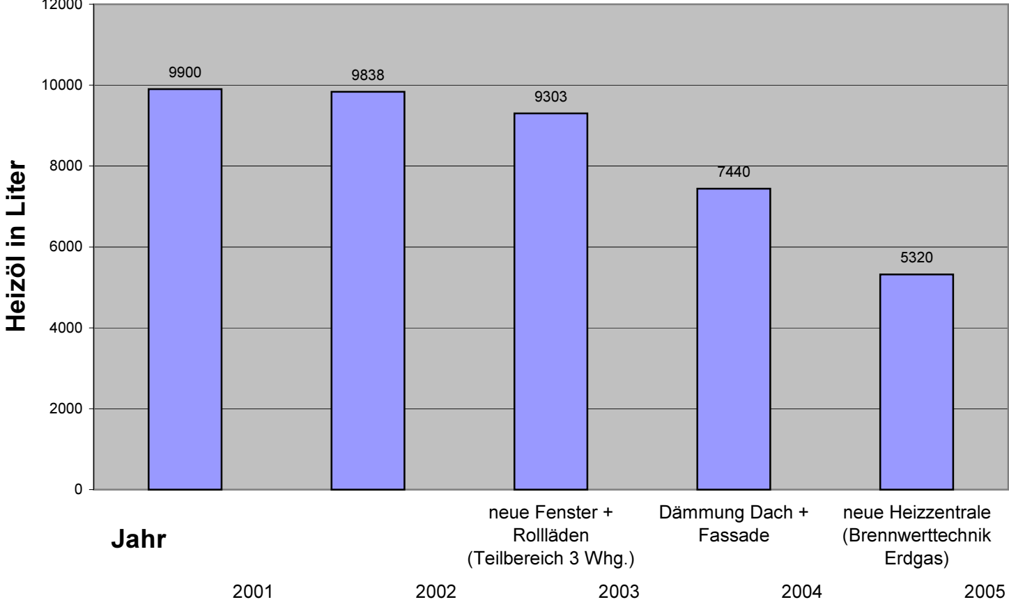
Auswirkung Energieeinsparmaßnahmen auf den Heizölverbrauch am Bsp. 6Fam.-Whs in Diedesheim
